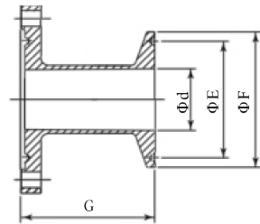
卡箍式接头 (HAB25~125, HDB15~125, HKB15~125)
