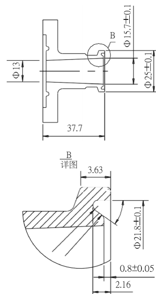
卡箍式接头 (HAB15)
