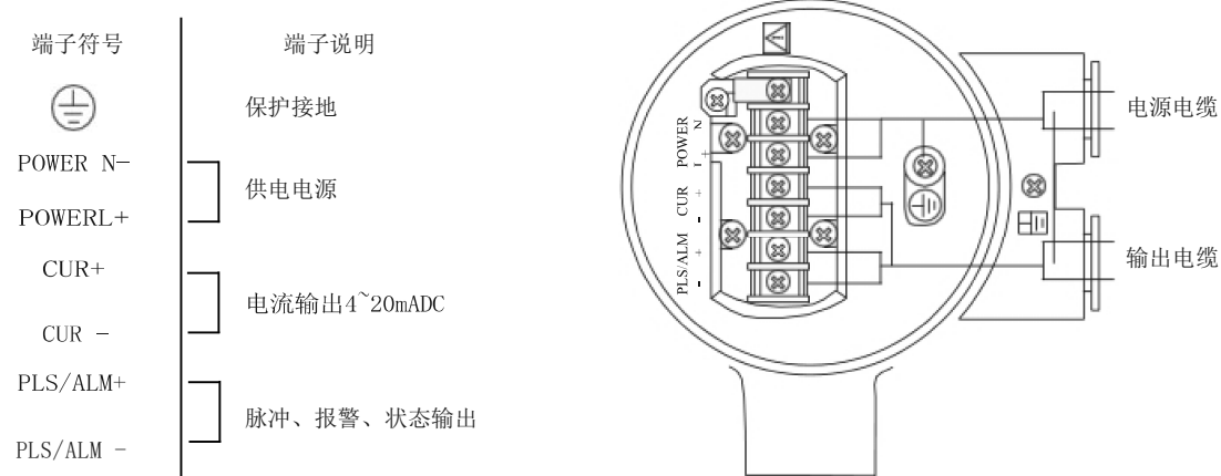
一体型接线端子示意图
