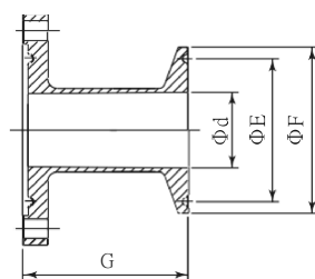
卡箍式接头 (HAB25~125,HDB15~125,HKB15~125)
