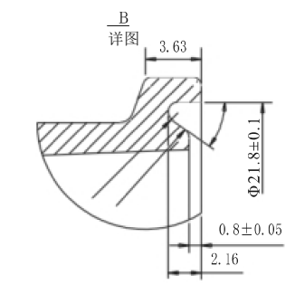
卡箍式接头 (HAB15)
